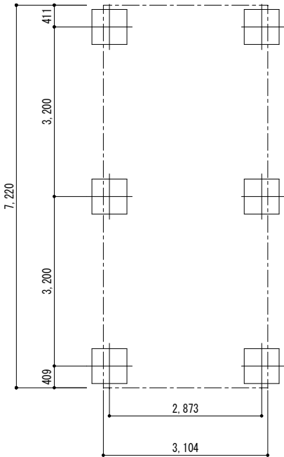
■ 基礎配置図
