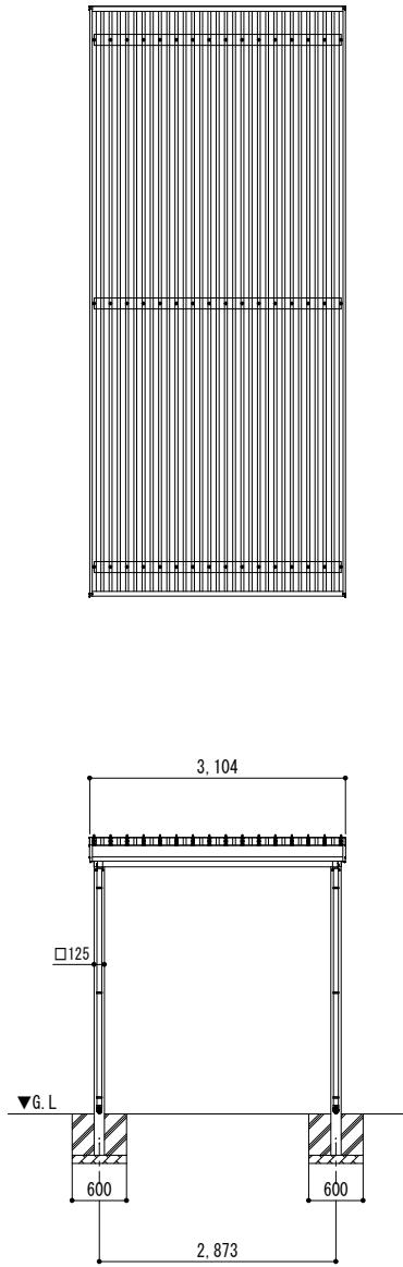
■ 姿図
